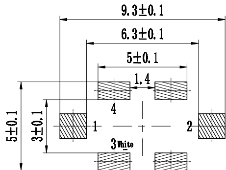
元件面孔位图
